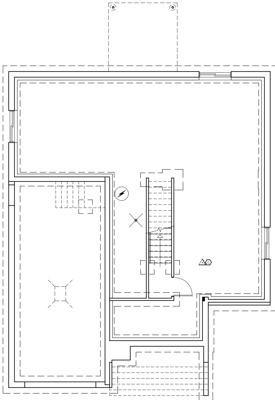
PLAN DES FONDATIONS
